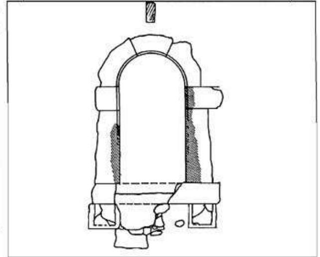
GVOZDANSKO, DOVRATNIK ULAZA U BRANIČ-KULU NA DRUGOM KATU (SKICA; ŠRAFATUROM SU OZNAČENA OŠTEĆENJA KAMENA)
