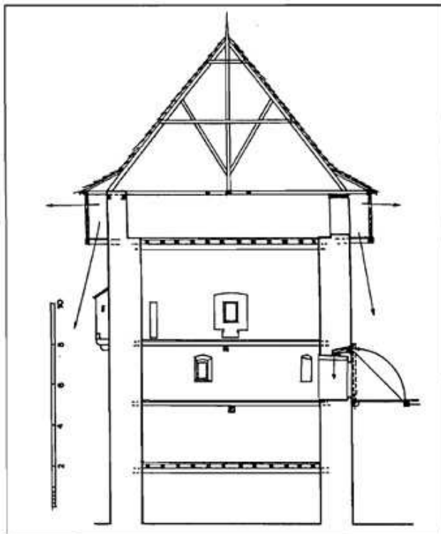
GVOZDANSKO, PRESJEK KROZ BRANIČ-KULU (SVE DRVENE KONSTRUKCIJE I ZAHOD NA KAMENIM KONZOLAMA PRETPOSTAVLJENI SU)
