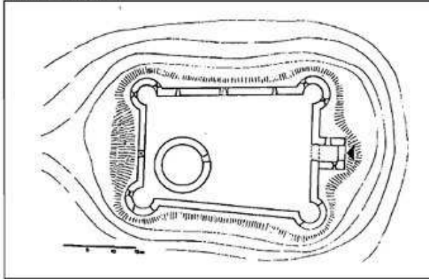
GVOZDANSKO, TLOCRT KAŠTELA U RAZINI PRIZEMLJA, SNIMKA OD PRIJE 14 GODINA)
